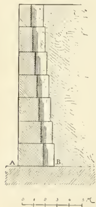
45. — Palais de Sargon. Coupe du mur, suivant AB. Place, t. III, pl. 35.
